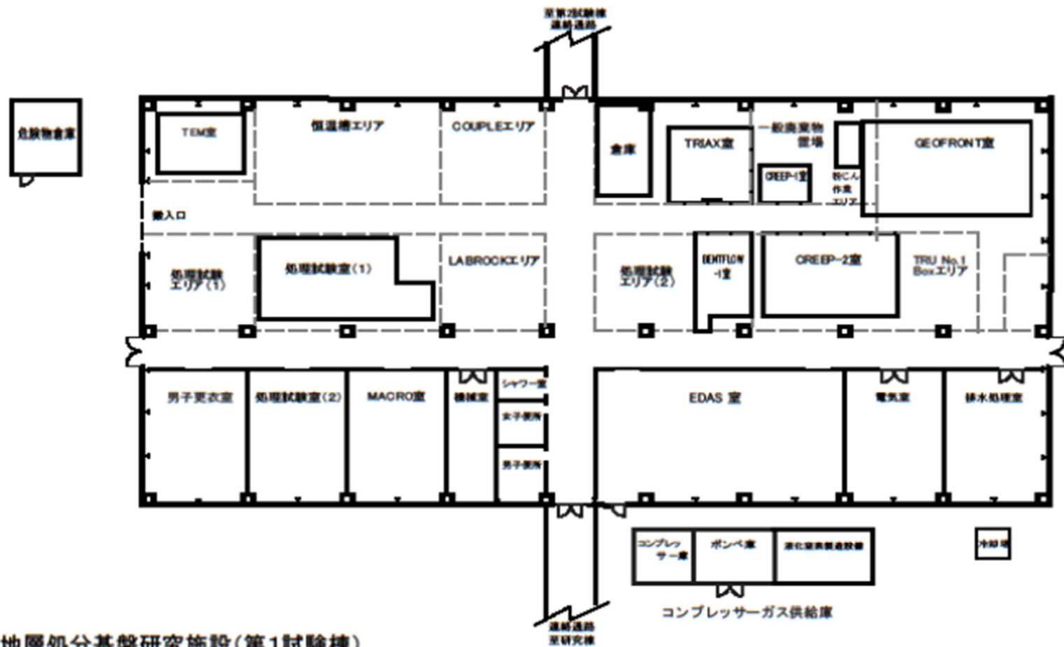
地層処分基盤研究施設(第1試験棟)
